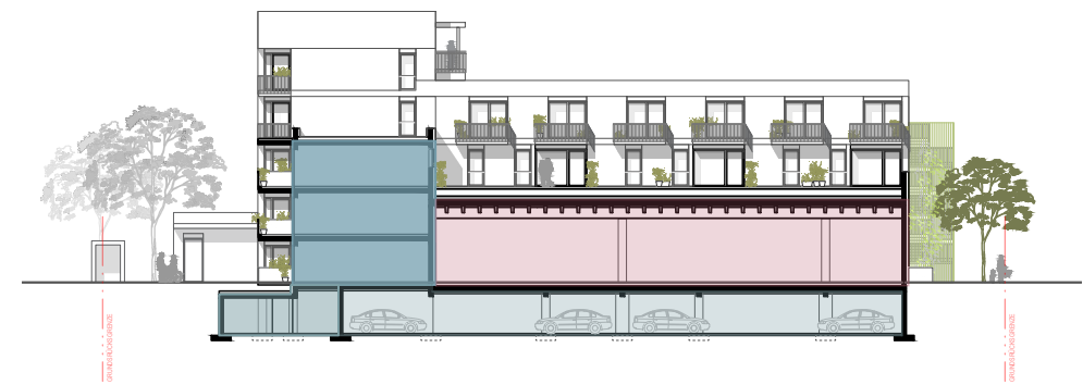
Schnitt D-D
