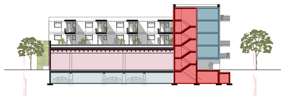
Schnitt E-E
